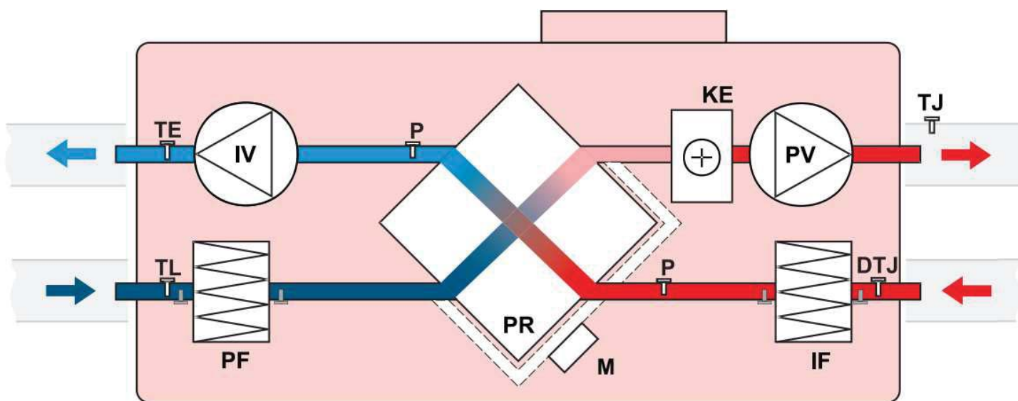
Tribwerk X-TYPE 1400 CE (вид со стороны обслуживания)
